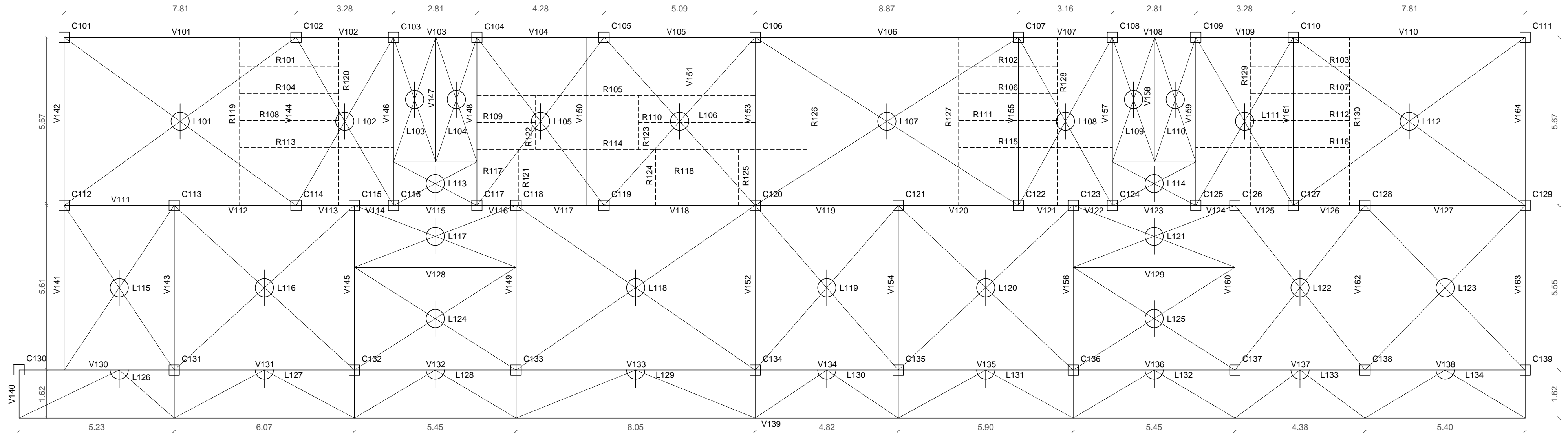
ESQUEMA ESTRUCTURAL SOBRE PLANTA BAJA
