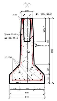
CORTE A-A
