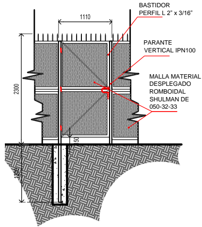
VISTA PORTÓN DE ACCESO PARA MANTENIMIENTO
